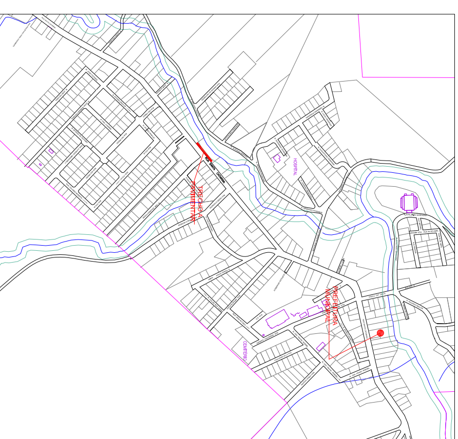
PLANTA DE LOCAÇÃO/SITUAÇÃO SEMI ESCALA
