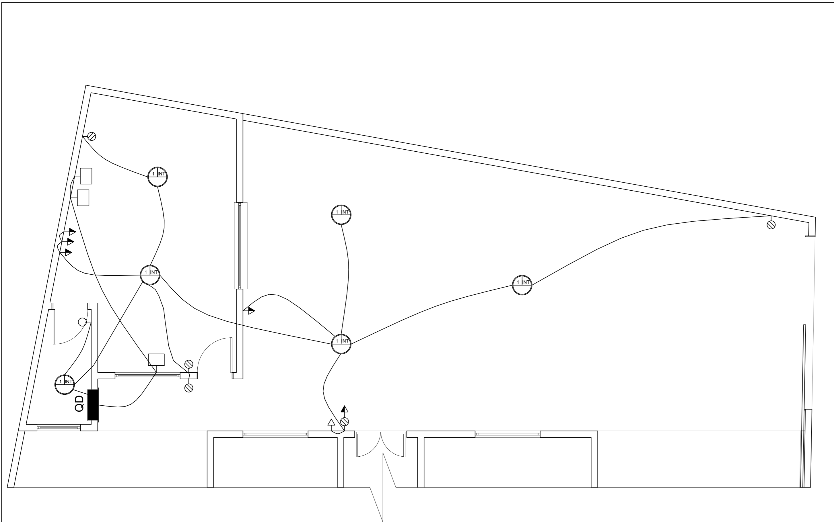
INSTALAÇÕES ELÉTRICAS Esc: 1/50
