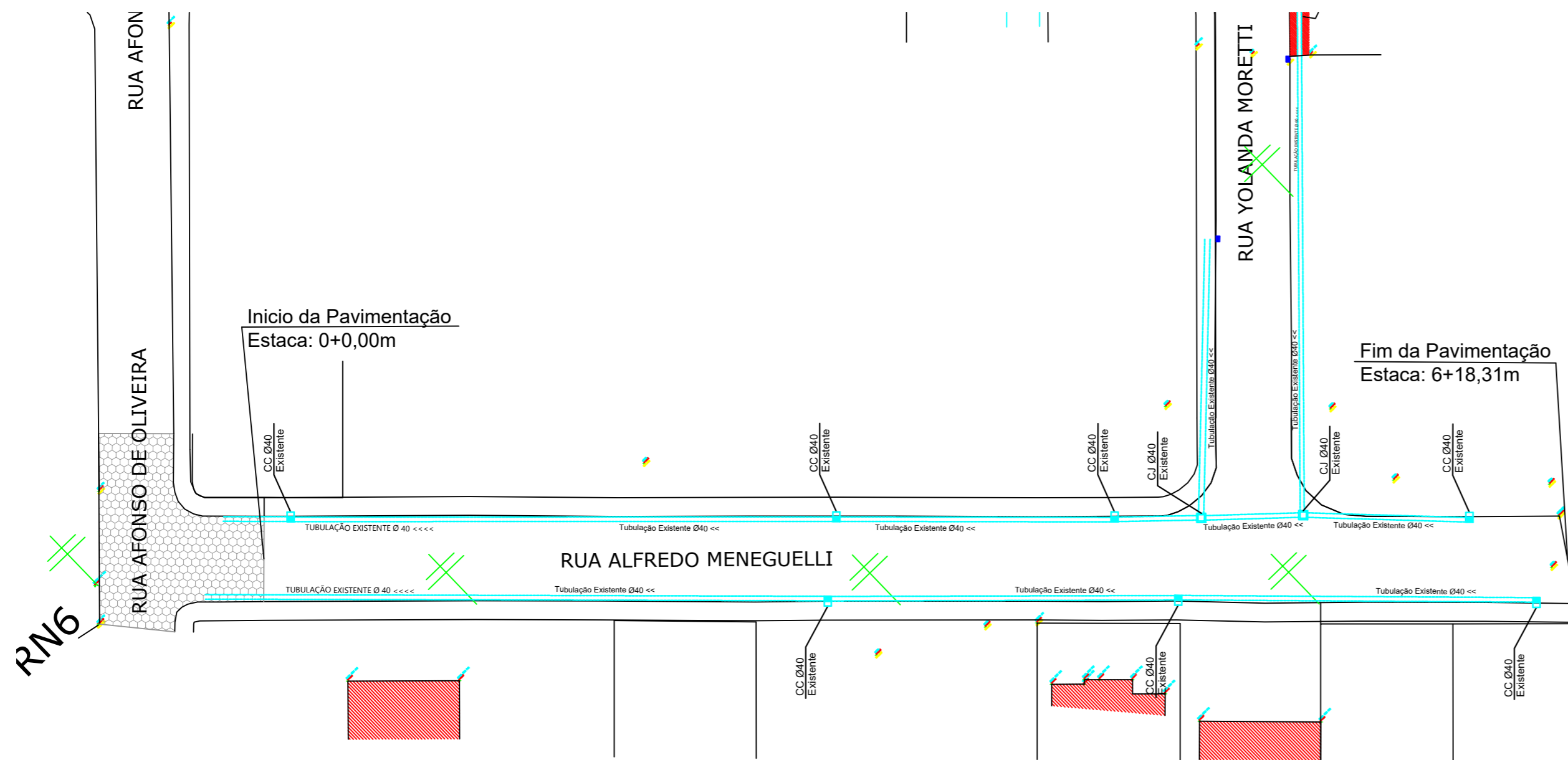
PLANTA DA DRENAGEM EXISTENTE ESC 1/500
