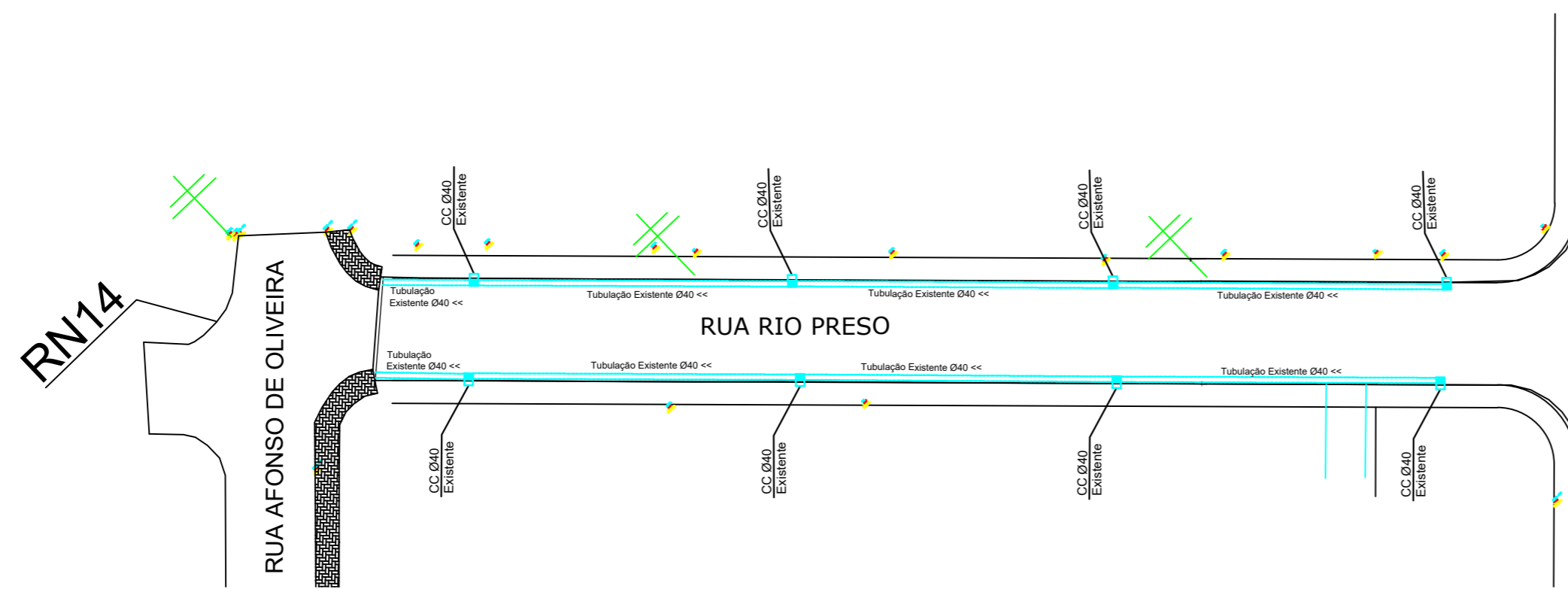
PLANTA DA DRENAGEM EXISTENTE ESC 1/500
