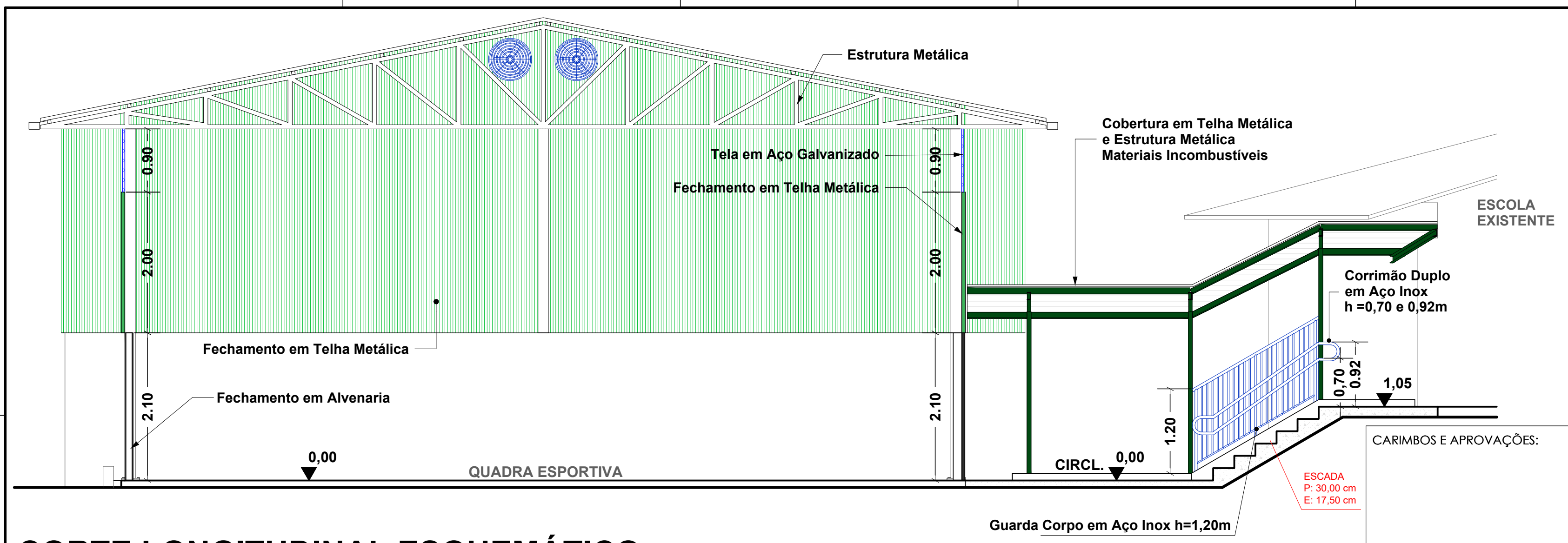
CORTE LONGITUDINAL ESQUEMÁTICO ESC: 1/50
