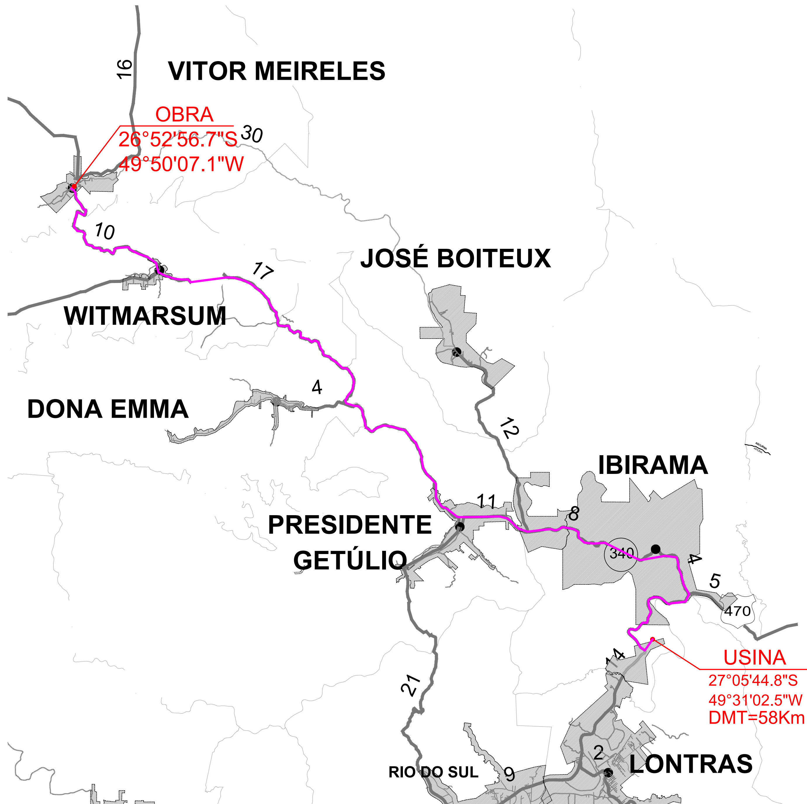
MAPA USINA DE ASFALTO SEM ESCALA
