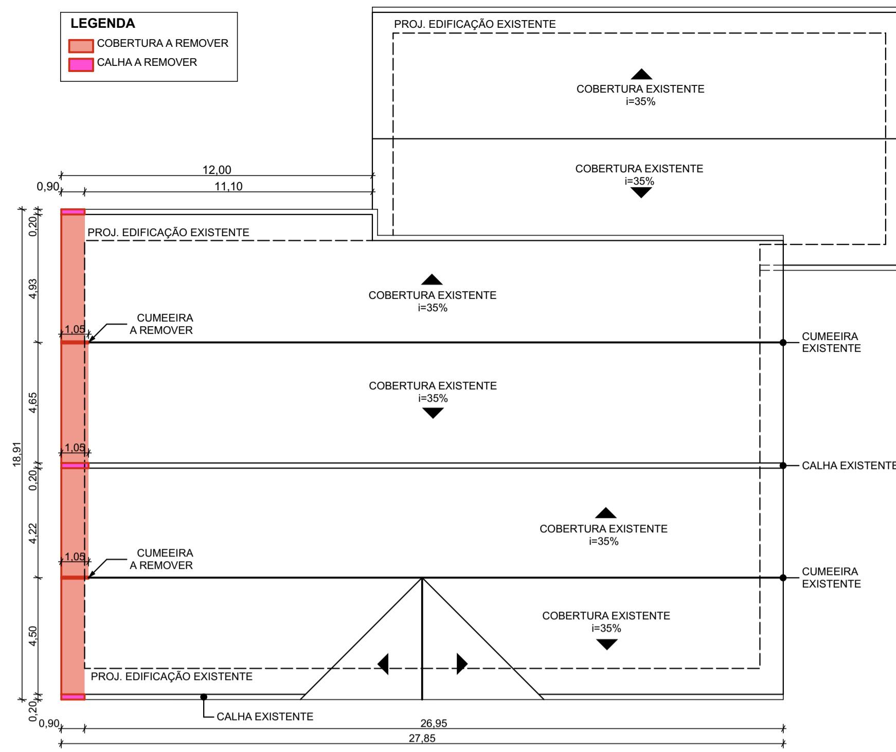
PLANTA DE DEMOLIÇÃO DA COBERTURA ESC.: 1/150
